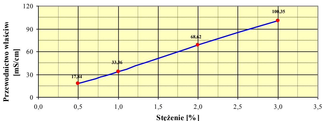
Wykres zależności przewodnictwa właściwego od stężania preparatu ORKAN FORTE
